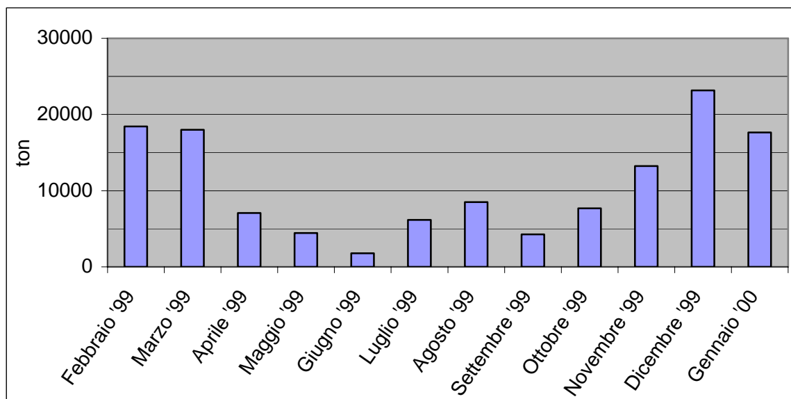
Figura 4. Traffico mensile GPL (transito per la biconca di Voltagrmana)
