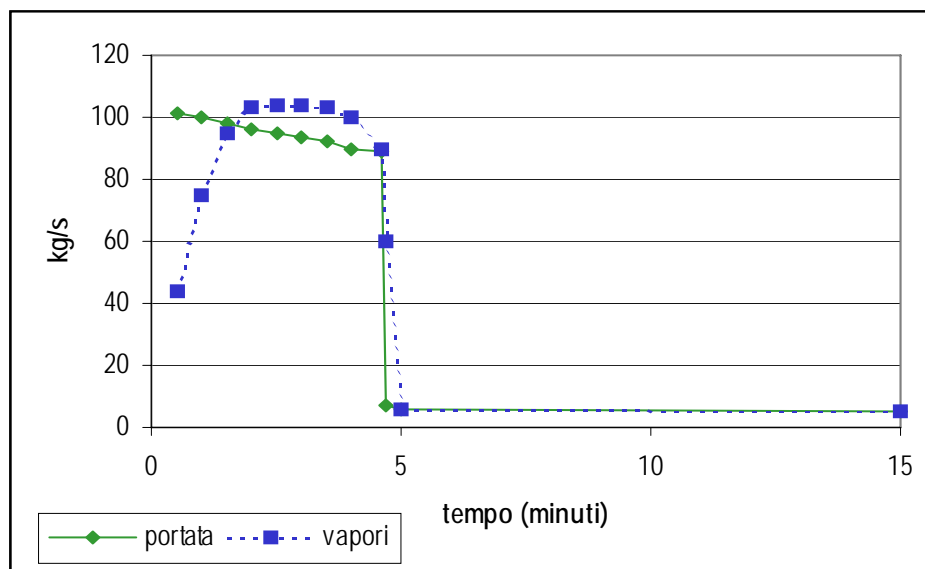
Figura 7. Andamento portata di efflusso ed evaporazione per ipotesi di collisione.
