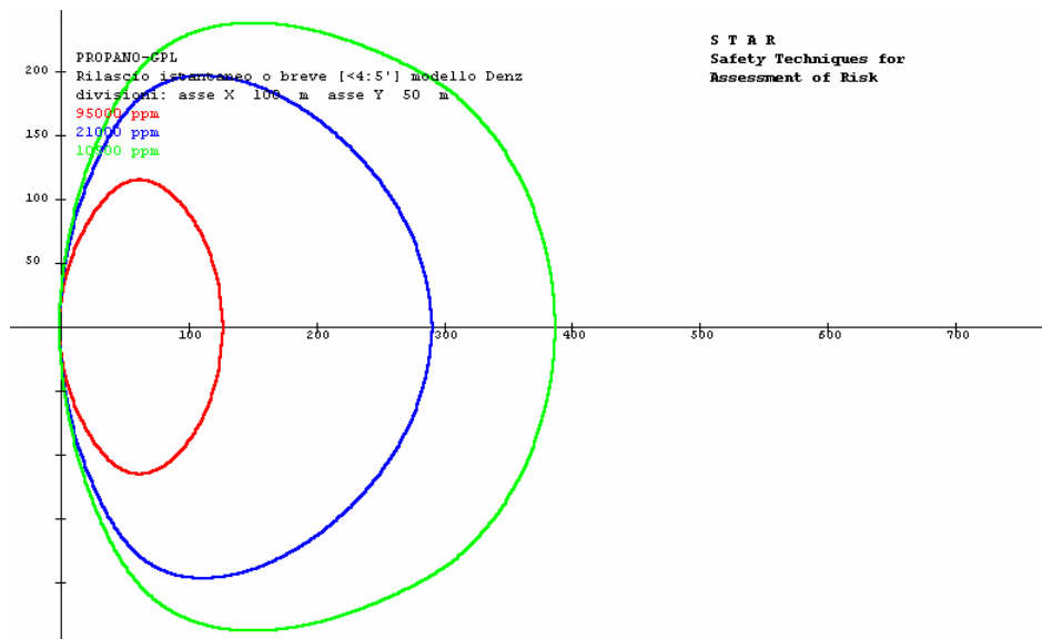
Figura 8. Scenario dispersione a seguito di collisione con rilascio
