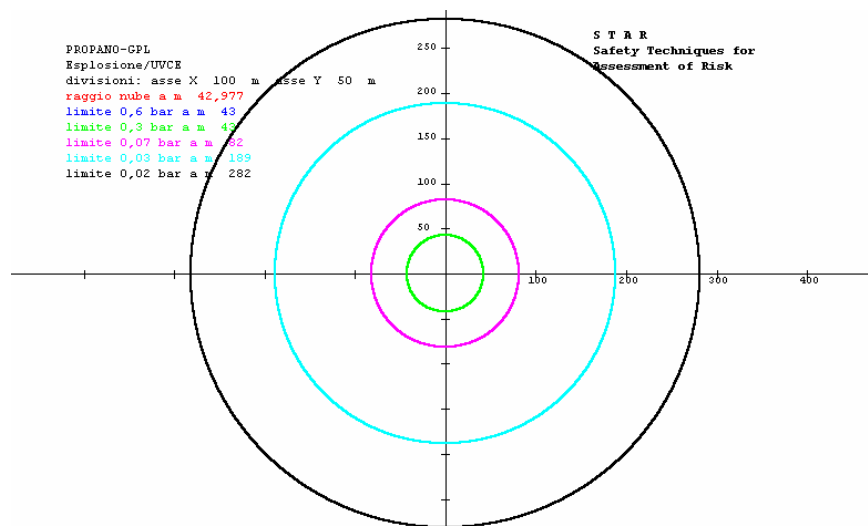
Figura 9. Scenario UVCE a seguito di collisione con rilascio.
