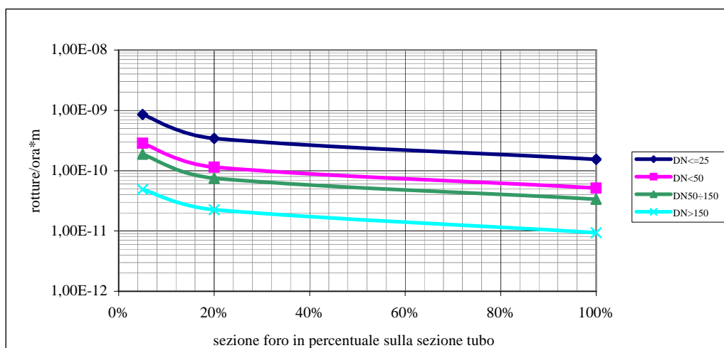
Figura 6. Frequenza attesa di rottura tubazioni (Lees 1996)
